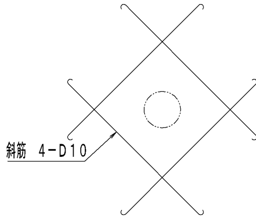
土間コンクリート補強図
