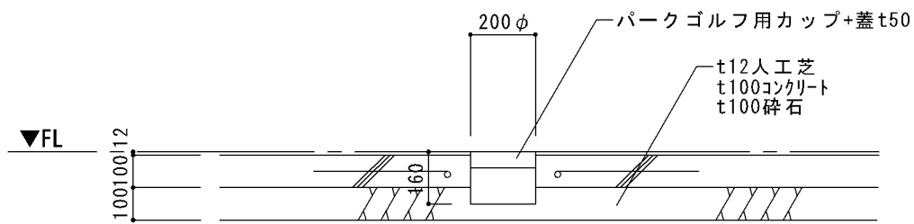
パークゴルフ用カップ詳細図
