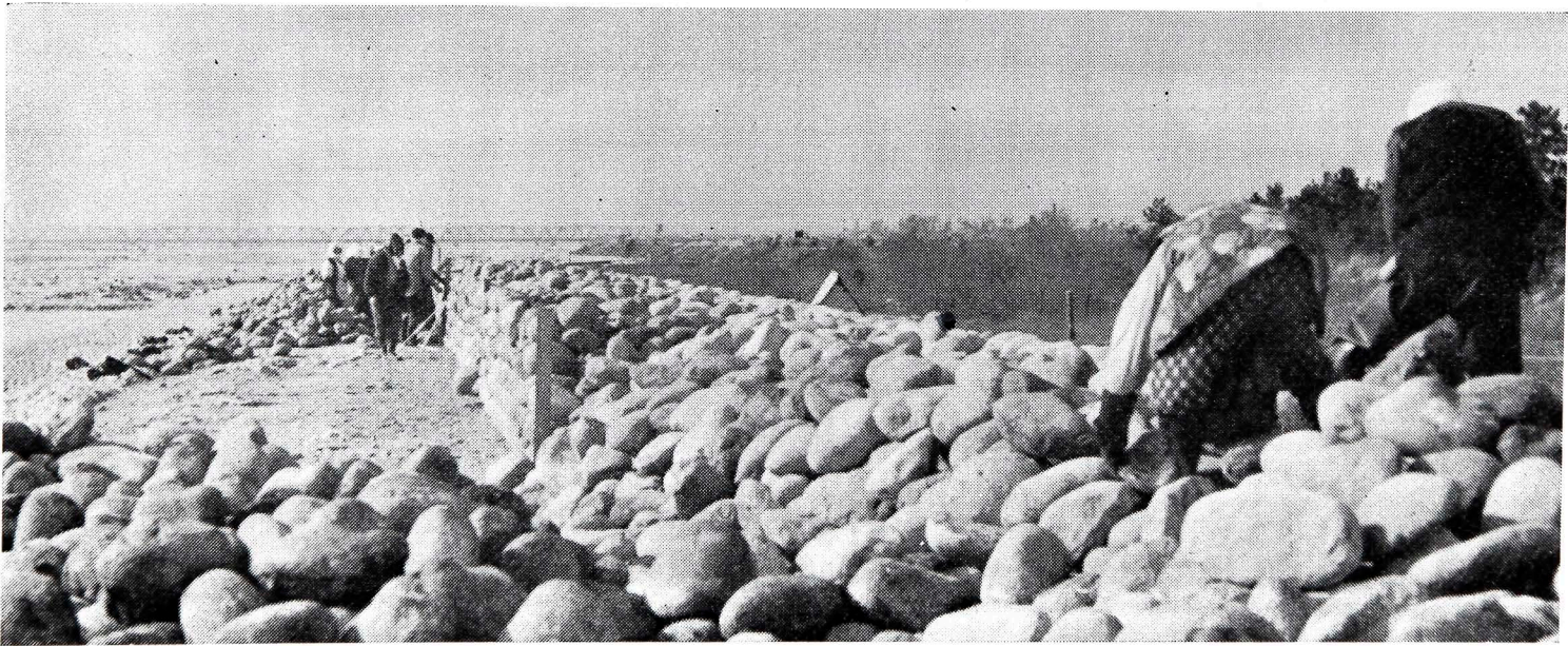
写真は黒部川右岸板屋地内でのため石整理作業(2月23日)
