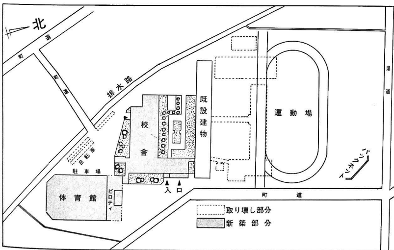
入善中学校増改築計画図
