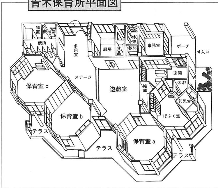
青木保育所平面図
