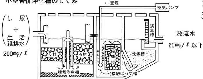
小型合併浄化槽のしくみ
