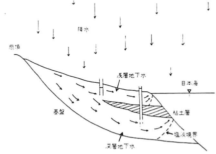
(図1) 黒部川扇状地における地質の断面模式図
