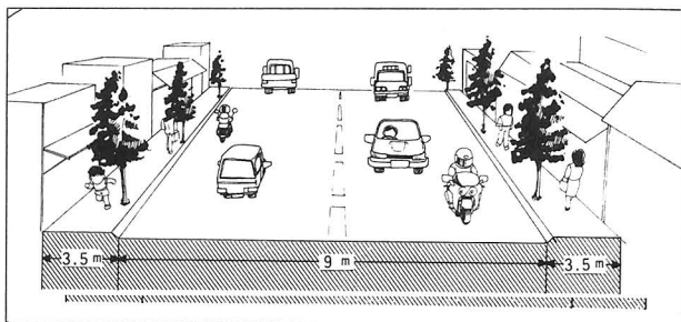
▼ 中央通り線の標準断面図
