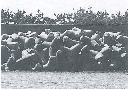
▲直立堤と消波工
