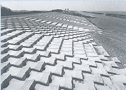
▲緩傾斜ブロック堤
