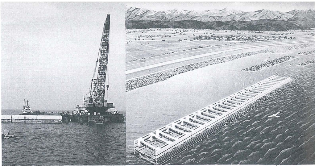
▲大型クレーン船を使った工事の様子
