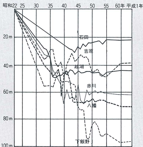
グラフ① 下新川海岸の汀線後退状況
