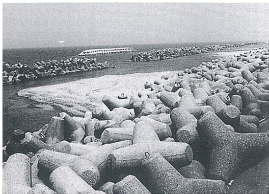
▲離岸堤、副離岸堤によって少しずつ育つたトンボロ(砂州)
