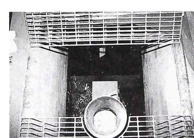
最終沈殿池を経てきれいになった水を、塩素混和池で細菌を消毒して放流する。
