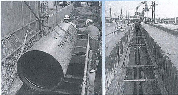
道路の下に埋められる下水管
