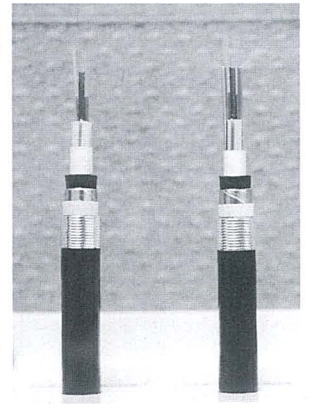
下水道管路に設置される光ファイバー
