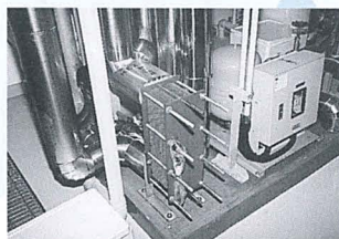
深層水活用施設の冷房用熱交換器
